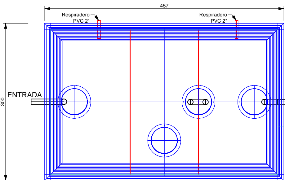
Tanque Séptico con Deflectores TSD-15 000
