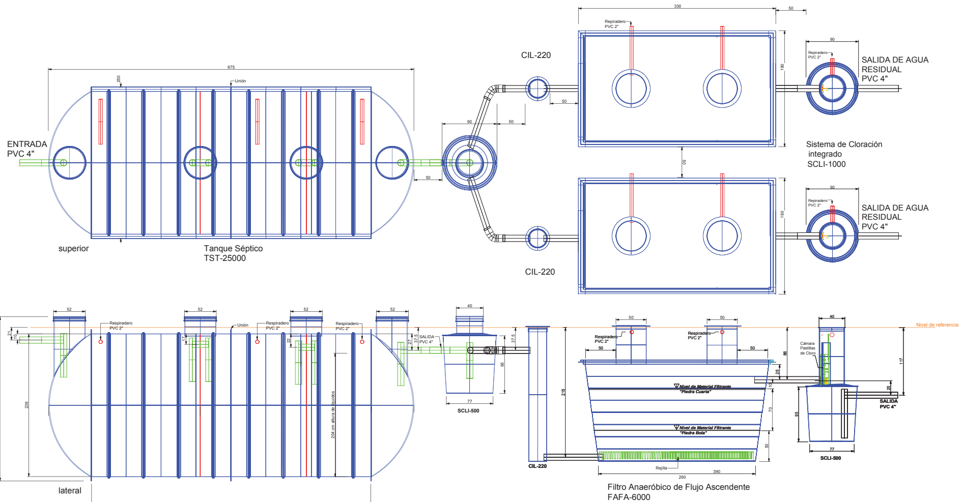
Tanque Séptico TST-25000
